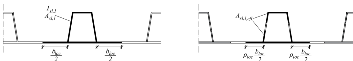
Figure 13. Longitudinal stiffener with adjacent parts of the plate for a) gross and b) effective cross section Slika 13. Vzdolžna ojačitev s sodelujočim delom pločevine za a) bruto in b) efektivni prerez
