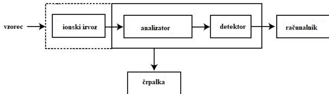
Slika 3: Shema masnega spektrometra
