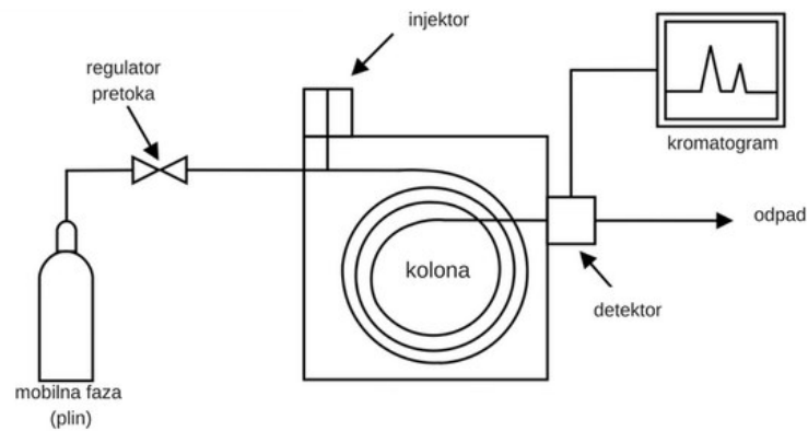
Slika 1: Shema plinskega kromatografa
