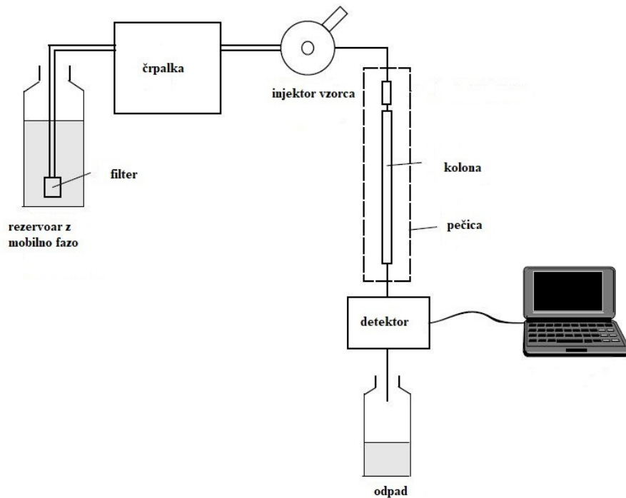
Slika 2: Shema tekočinskega kromatografa
