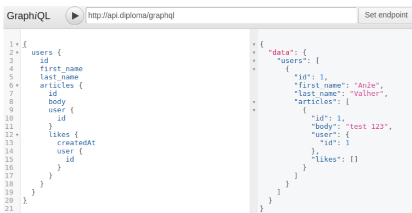
Slika 4.7: Primer poizvedbe.
