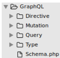
Slika 4.5: Struktura imenikov.
