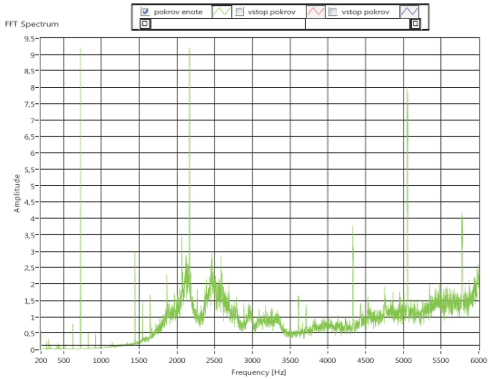
Slika 7.1: Amplitudna analiza vibracij na vstopu s togim pokrovom- mikrofoni 2
