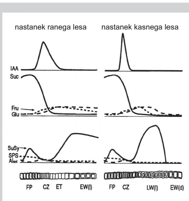
□ Slika 1. Shematski prikaz porazdelitve avksina, karbohidratov in aktivnosti saharoznih presnovnih encimov v kambiju, diferencirajočih se in zrelih derivatih ranega in kasnega lesa (Uggla in sod., 2001). FP – floemske celice, Suc – saharozna, Fru – fruktoza, Glu – gluktoza, SuSy – saharozna sintaza, SPS – Suc-fosfatna sintaza, Al – kislinjska invertaza, FP – floem, CZ – kambij, ET – traheide v postkambijski rasti, EW (l) – traheide ranega lesa v procesu odlaganja sekundarne celične stene in lignifikacije, EW(d) – zrele traheide, LW(l) – traheide kasnega lesa v procesu odlaganja sekundarne celične stene in lignifikacije
